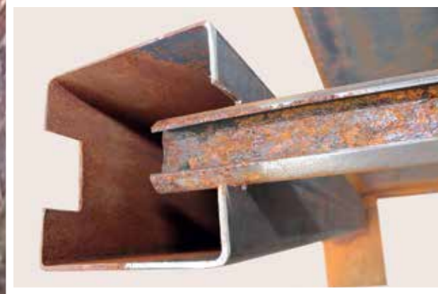
Mit der Fixierleiste können die Zaunpfosten ausgerichtet werden.
