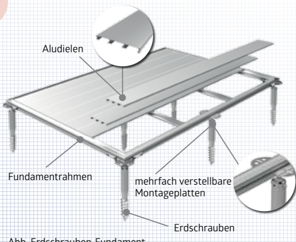
Abb. Erdschrauben-Fundament
